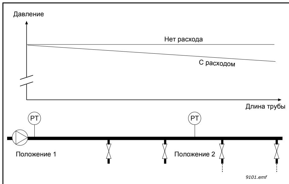
Рис. 93. Размещение датчика давления (PT)
