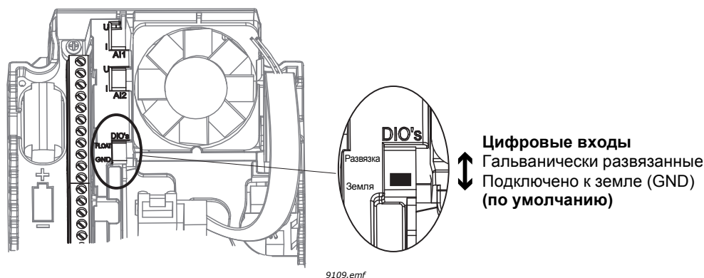
Рис. 107. DIP-переключатель изоляции
