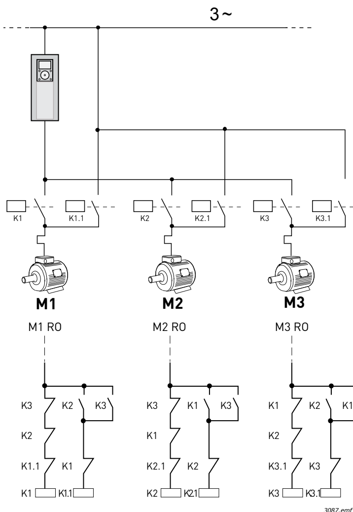
Рис. 109. M1-3 RO = управление двигателем от реле
