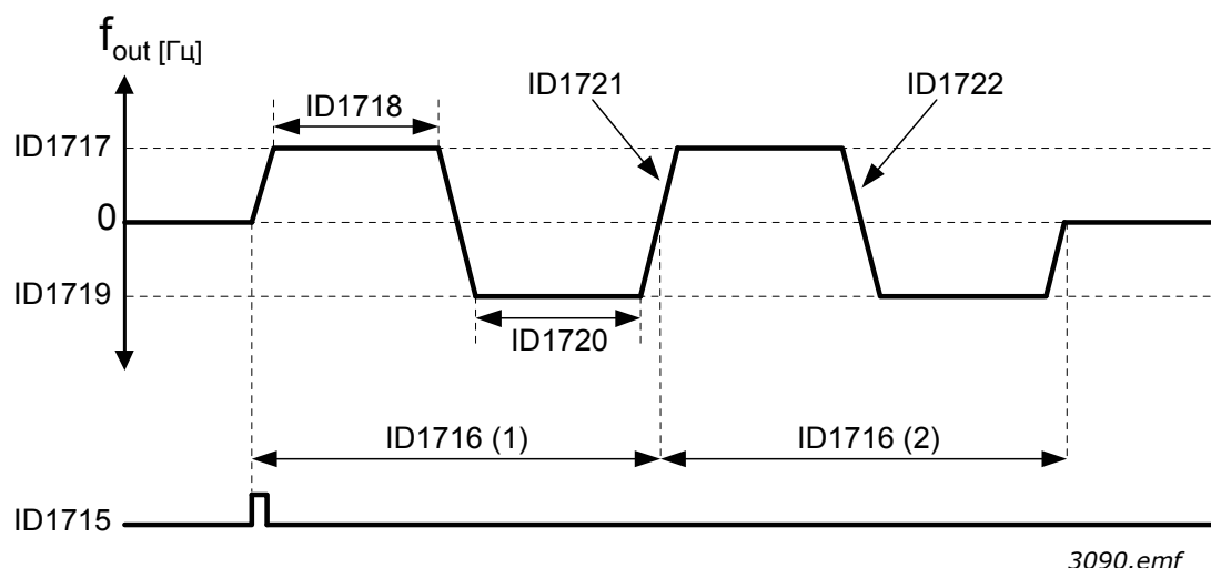
Рис. 115. Функция автоматической очистки. (0 = нулевая частота, ID 1716 = циклы очистки 1 и 2), ID 1715 = P3.5.1.41 Активизация автоматической очистки, ID 1717 = P3.21.1.8 Частота очистки в прямом направлении, ID 1718 = P3.21.1.9 Время очистки в прямом направлении, ID 1719 = P3.21.1.10 Частота очистки в обратном направлении, ID 1720 = P3.21.1.11 Время очистки в обратном направлении, ID 1721 = P3.21.1.12 Время разгона при очистке, ID 1722 = P3.21.1.13 Время замедления при очистке
