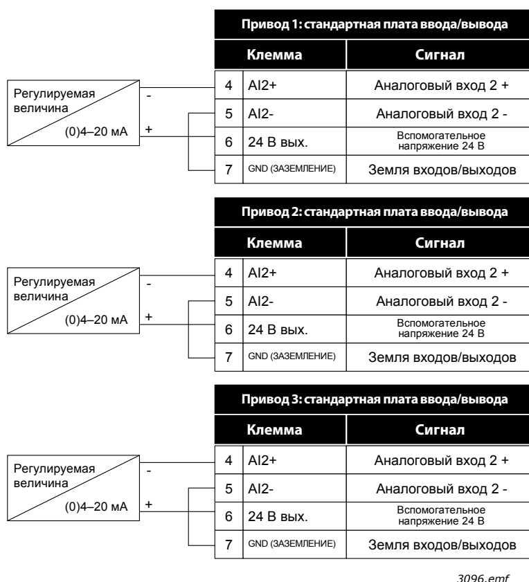
Рис. 104. Принцип подключения отдельных датчиков обратной связи
