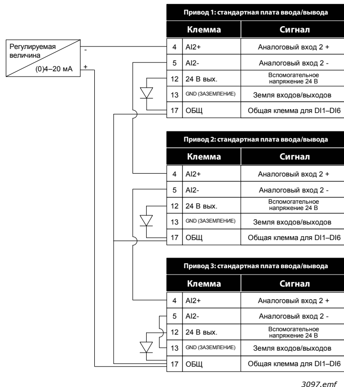
Рис. 105. Принцип подключения общего датчика (питание от платы ввода-вывода привода)
