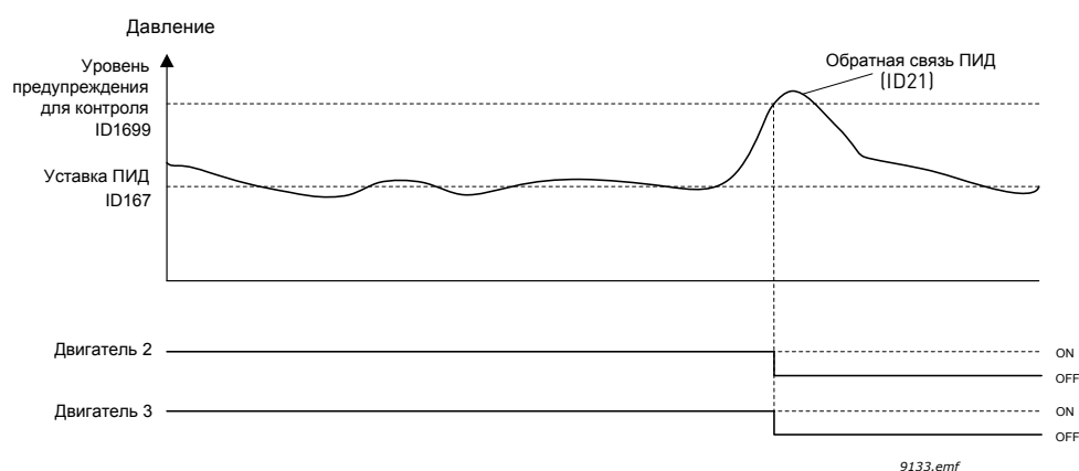
Рис. 111. Контроль избыточного давления
