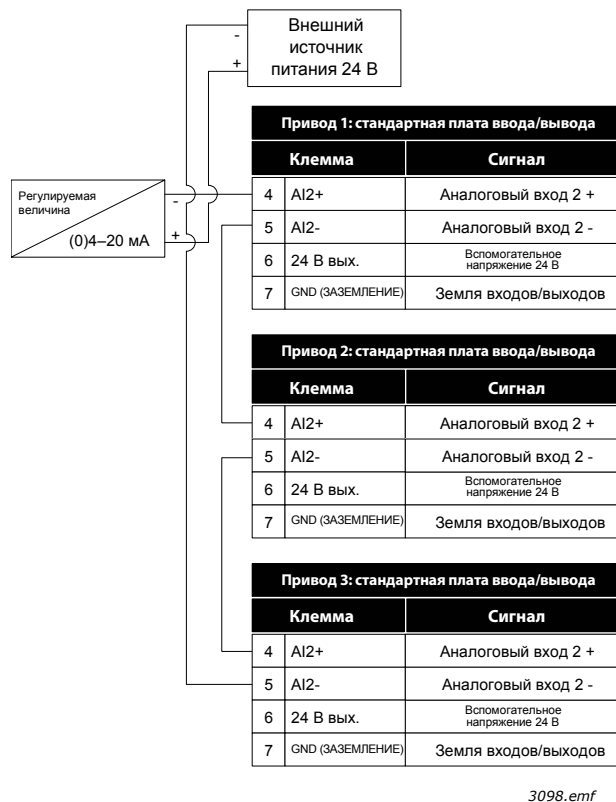
Рис. 106. Принцип подключения общего датчика (питание от внешнего источника напряжением 24 В)
