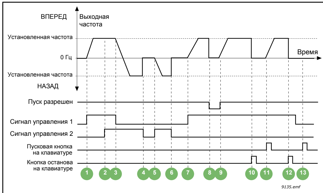
Рис. 53. Логика пуска/останова I/O A = 0
