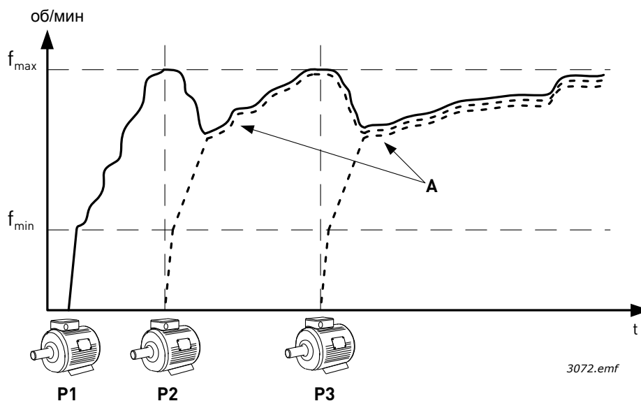
Рис. 102. Регулирование насоса в режиме с несколькими ведомыми насосами. Насос 1 является ведущим, скорость насосов 2 и 3 соответствует скорости насоса 1, как показано кривыми А.
