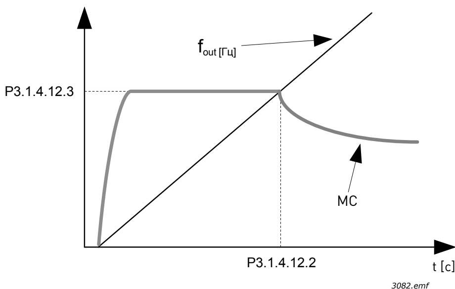
Рис. 51. Пуск I/f (MC = ток двигателя), P3.1.4.12.2 = Частота пуска I/f, P3.1.4.12.3 = Пусковой ток I/f
