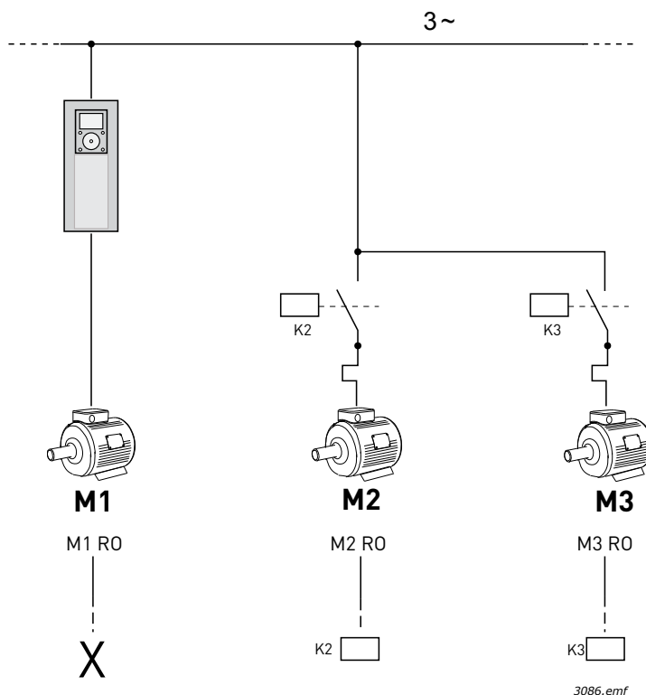
Рис. 108. M1-3 RO = Управление двигателем от реле, X = не используется
