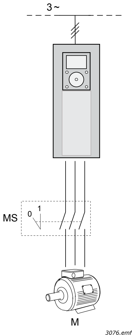
Рис. 47. Коммутатор двигателя
