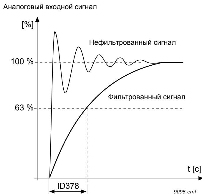
Рис. 68. Фильтрация сигнала А11
