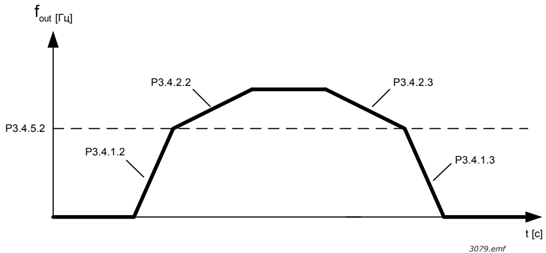
Рис. 60. Кривая 2 активируется, когда выходная частота превышает пороговый уровень. (P.3.4.5.2 = Пороговая частота кривой изменения скорости, P3.4.1.2 = Время ускорения 1, P3.4.2.2 = Время ускорения 2, P3.4.1.3 = Время замедления 1, P3.4.2.3 = Время замедления 2)
